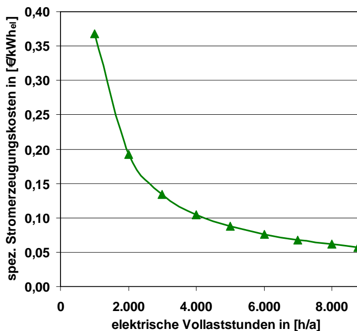
Abbildung 11: Spezifische Stromerzeugungskosten in Abhängigkeit der Anlagenauslastung (Jahresvollaststunden) - Biomasse-KWK-Anlage auf ORC-Basis (500 kW el )
