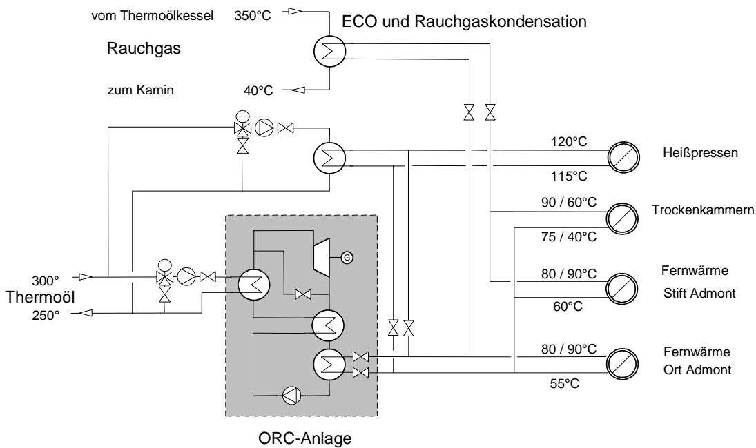
Abbildung 3: Einbindung des ORC-Prozesses in das Biomasse-Heizkraftwerk der Holzindustrie STIA/Admont
